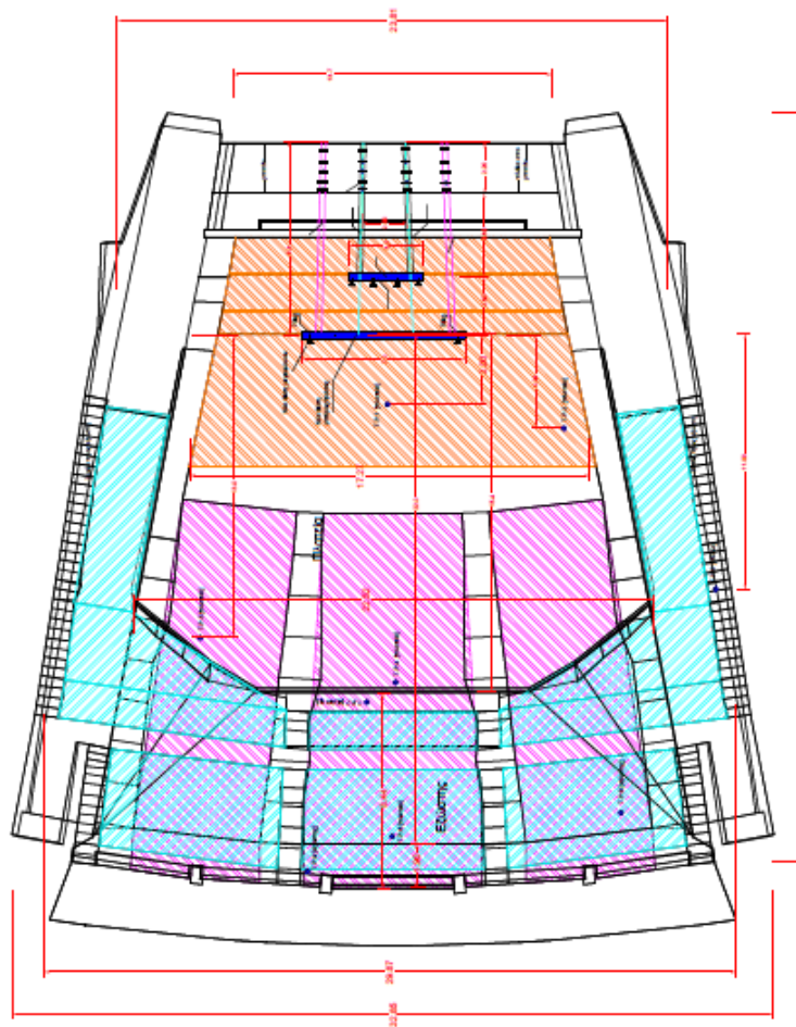
Σχέδιο Α (κάτοψη, θέση ηχείων)
