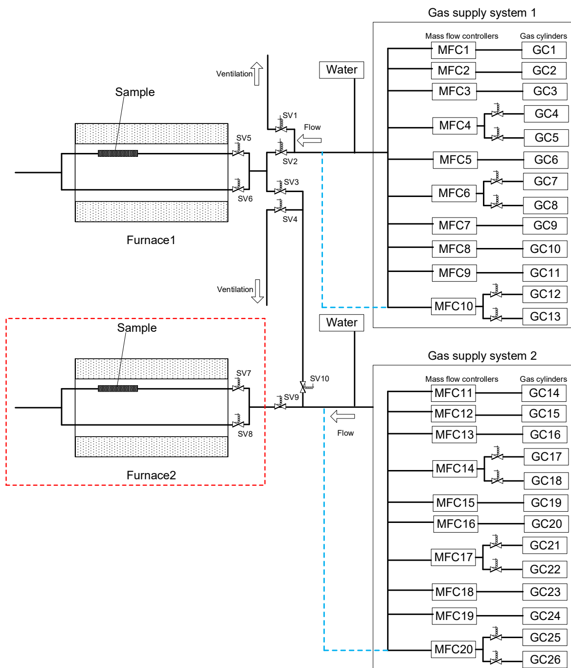
Εικόνα 1 Διάταξη ροής
