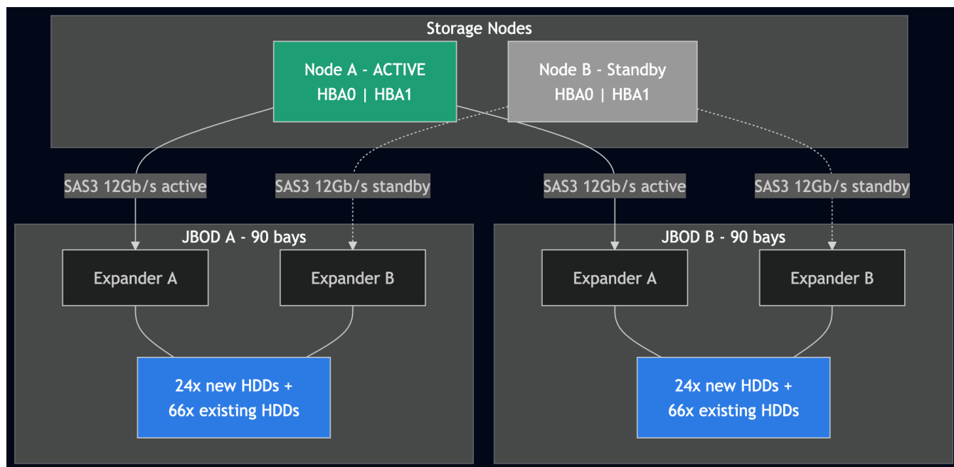
ΠΤΧ 3.1: Τεχνικά χαρακτηριστικά εξυπηρετητών αποθηκευτικού cluster
